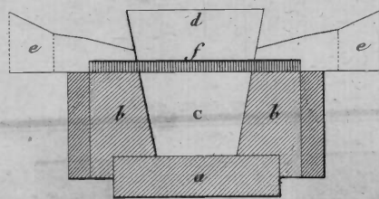
Fig. 6. Coupe suivant EF. de fig. 5.
